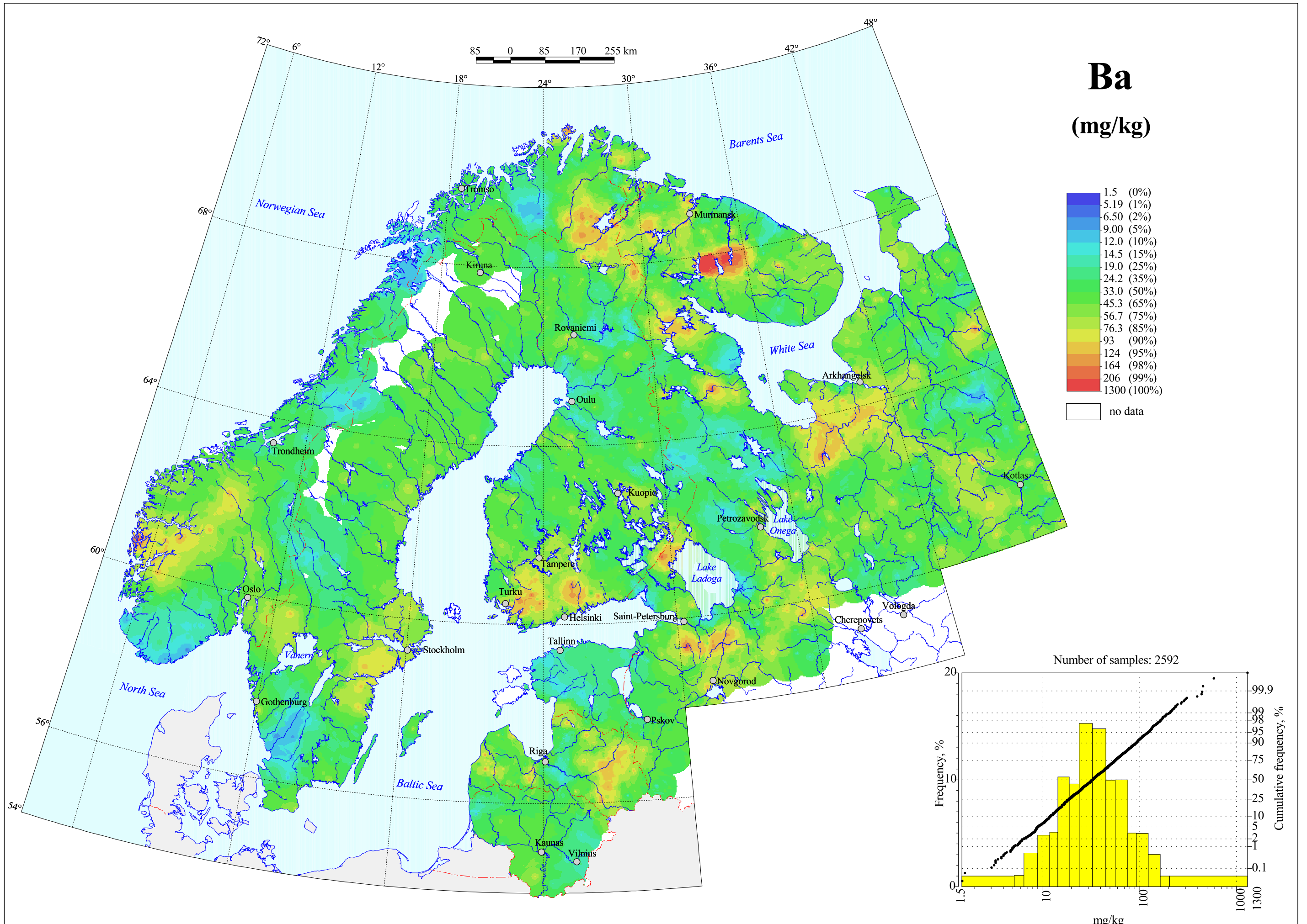
Barium in C-horizon, Grain Size <2 mm, Aqua regia Extraction
